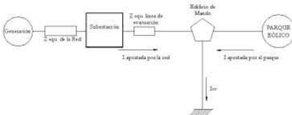
Figura 3: Esquema conceptual de un cortocircuito.
