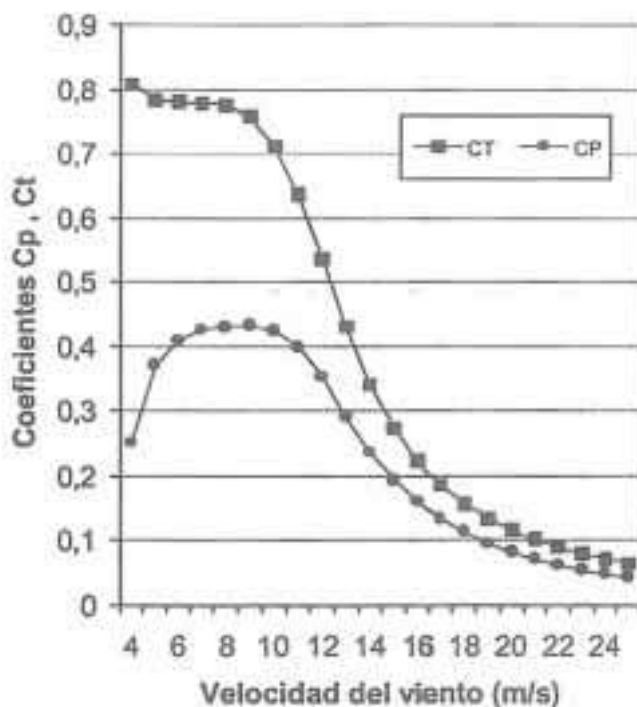
Figura 2: Curva de potencia.
