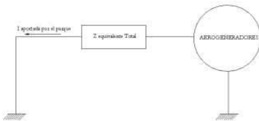
Figura 5: Esquema eléctrico del circuito de aportación de los aerogeneradores.
