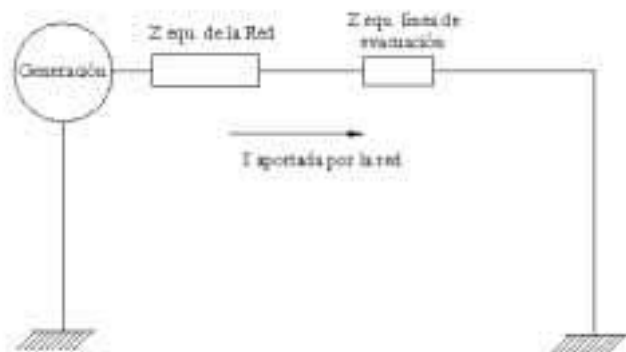
Figura 4: Esquema eléctrico del circuito de aportación a la red.
