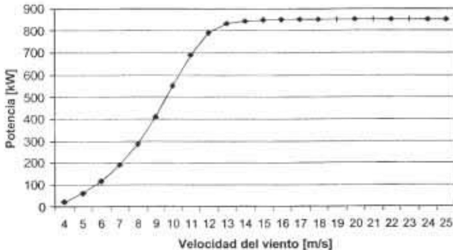
Figura 1: Curva de potencia.
